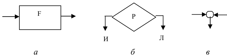
Рис. 1.1. Основные типы узлов в блок-схемах: а – функциональный, б – предикатный, в – слияния
