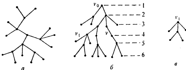
Рис. 8.4. Деревья: а – дерево; б – растущее дерево с корнем v_0 ; 1, 2, ..., 6 – уровни вершин; в – поддерево растущего дерева
