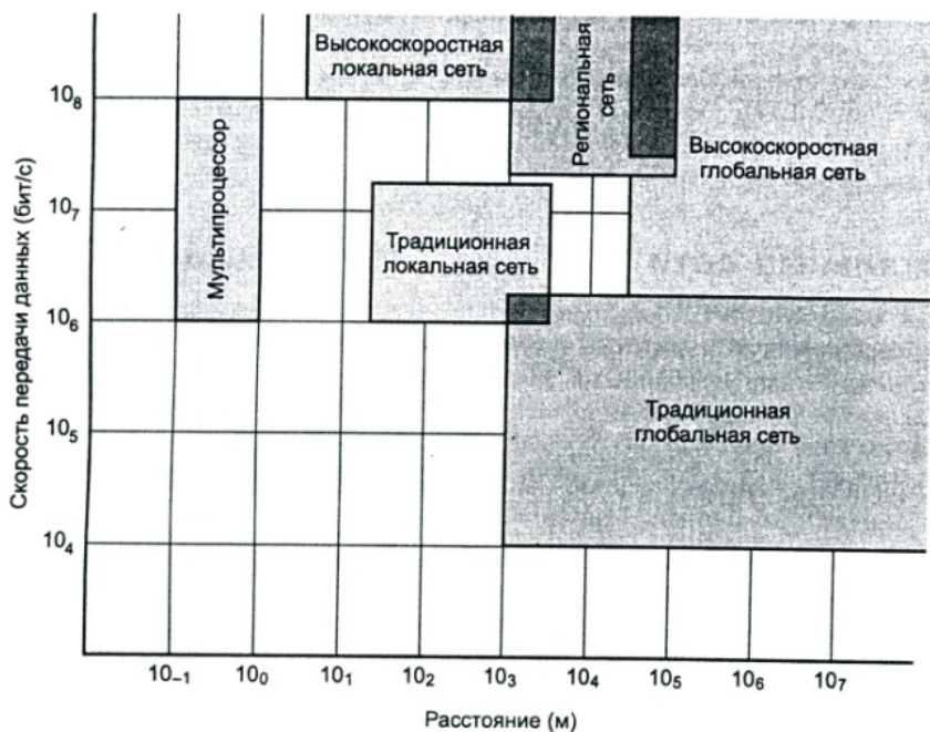
Рис. 4.22. Сравнение мультимплексных систем, а также локальных, региональных и глобальных сетей
