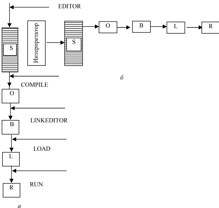
Рис. 6.5. Схема работы компилятора (a) и интерпретатора (б)
