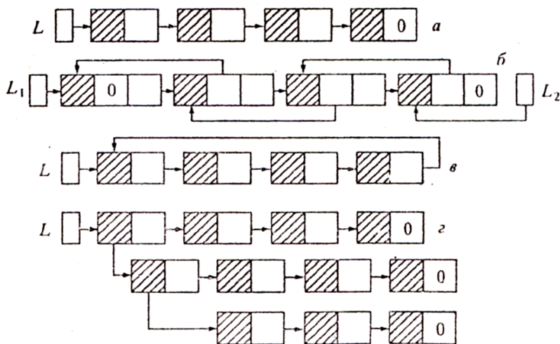
Рис. 8.2. Списки: a — однонаправленный; б — двунаправленный; в — кольцевой; г — иерархический; L , L 1 , L 2 — заголовки списков; информационное поле заштриховано
