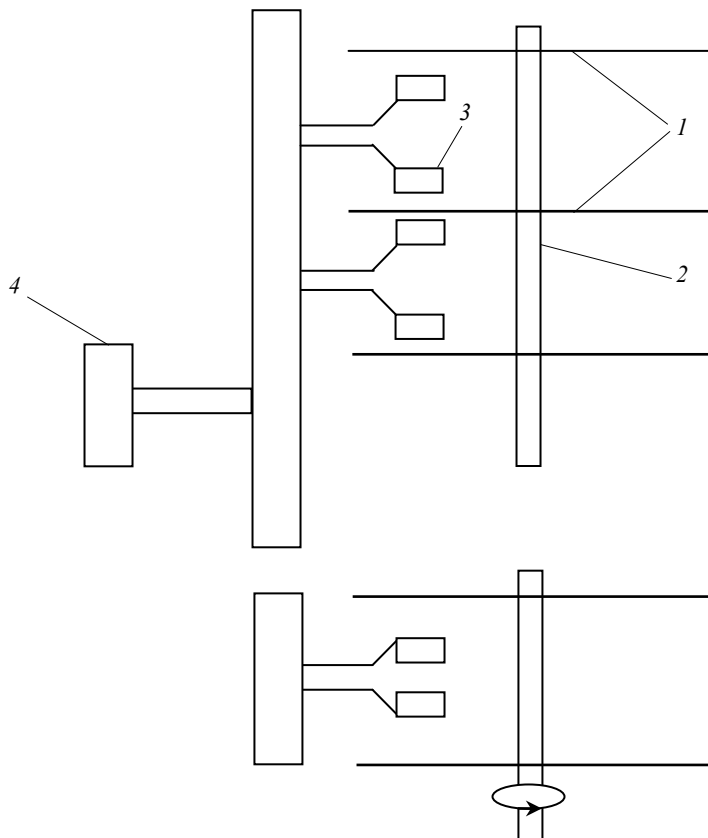
Рис. 2.7. Кинематическая схема накопителя на магнитном диске:
