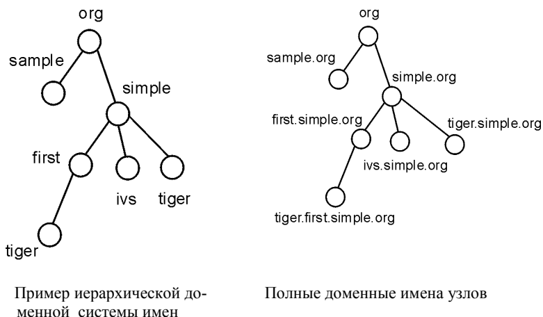
Рис. 4.15. Иерархия доменных имен
