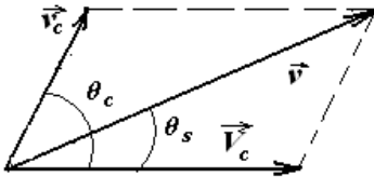
Рис. 3.14. Диаграмма скоростей нейтрона в разных системах координат
