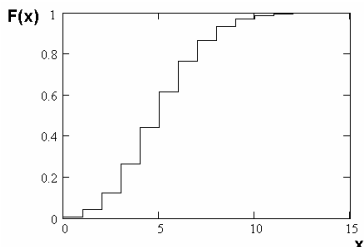
Рис. 3.4. График функции распределения Пуассона ( n=5 )
