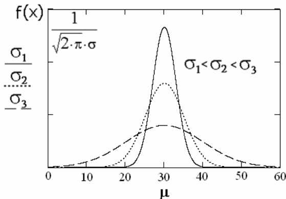
Рис. 3.1. График функции плотности нормального распределения для \mu = 30 и различных значений \sigma_1, \sigma_2 и \sigma_3
