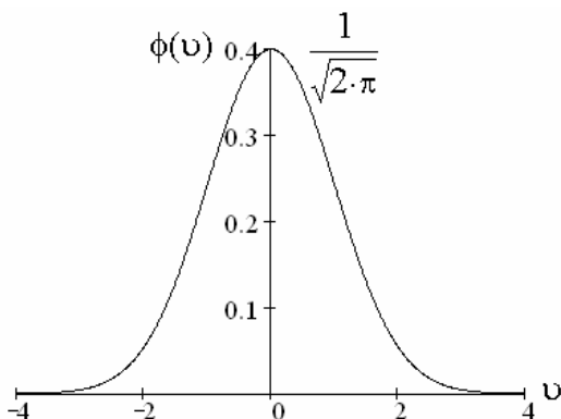
Рис. 3.2. График функции плотности вероятности стандартного нормального распределения
