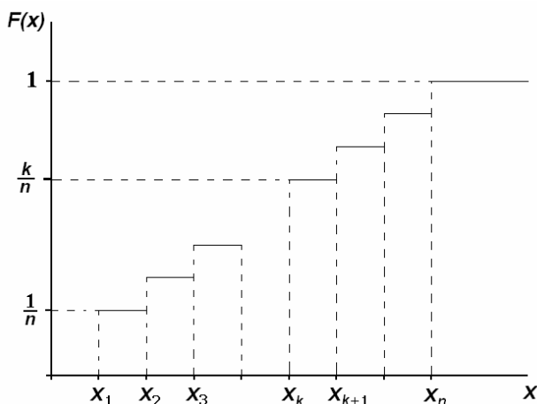
Рис. 6.1. График экспериментальной функции распределения вероятности
