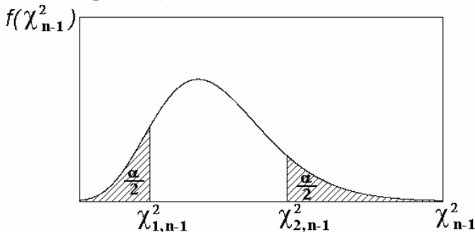
Рис. 4.1. График функции плотности вероятности для распределения \chi^2
