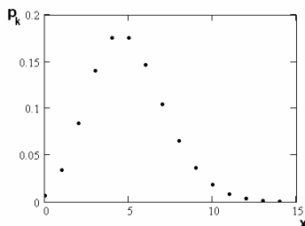
Рис. 3.5. График плотности функции распределения Пуассона ( n=5 )
