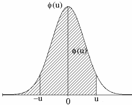
Рис. 3.3. График функции плотности стандартного нормального распределения.
